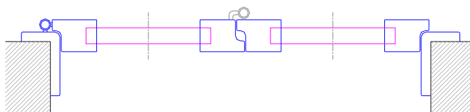
BIANTA RIBALTABILE SX TIPOLOGIA: BSX1
