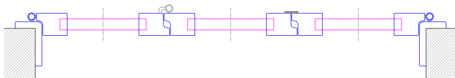
TRIANTA RIBALTABILE DX TIPOLOGIA: TDX1
