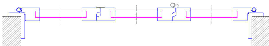
TRIANTA RIBALTABILE SX TIPOLOGIA: TSX1
