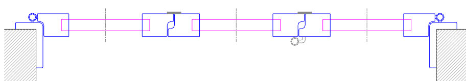
TRIANTA SNODATA SX TIPOLOGIA: TSX2
