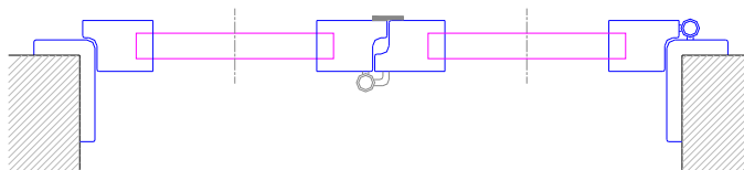
BIANTA SNODATA DX TIPOLOGIA: BDX2
